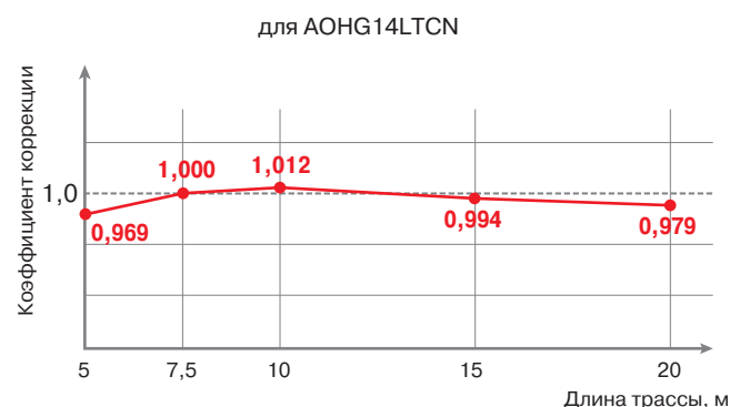
График коррекции теплопроизводительности в зависимости от длины трассы
