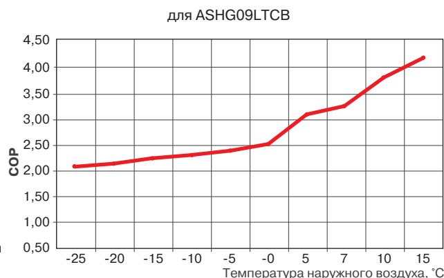
График изменения COP в зависимости от уличной температуры (при поддержании в помещении температуры 20 °C)
